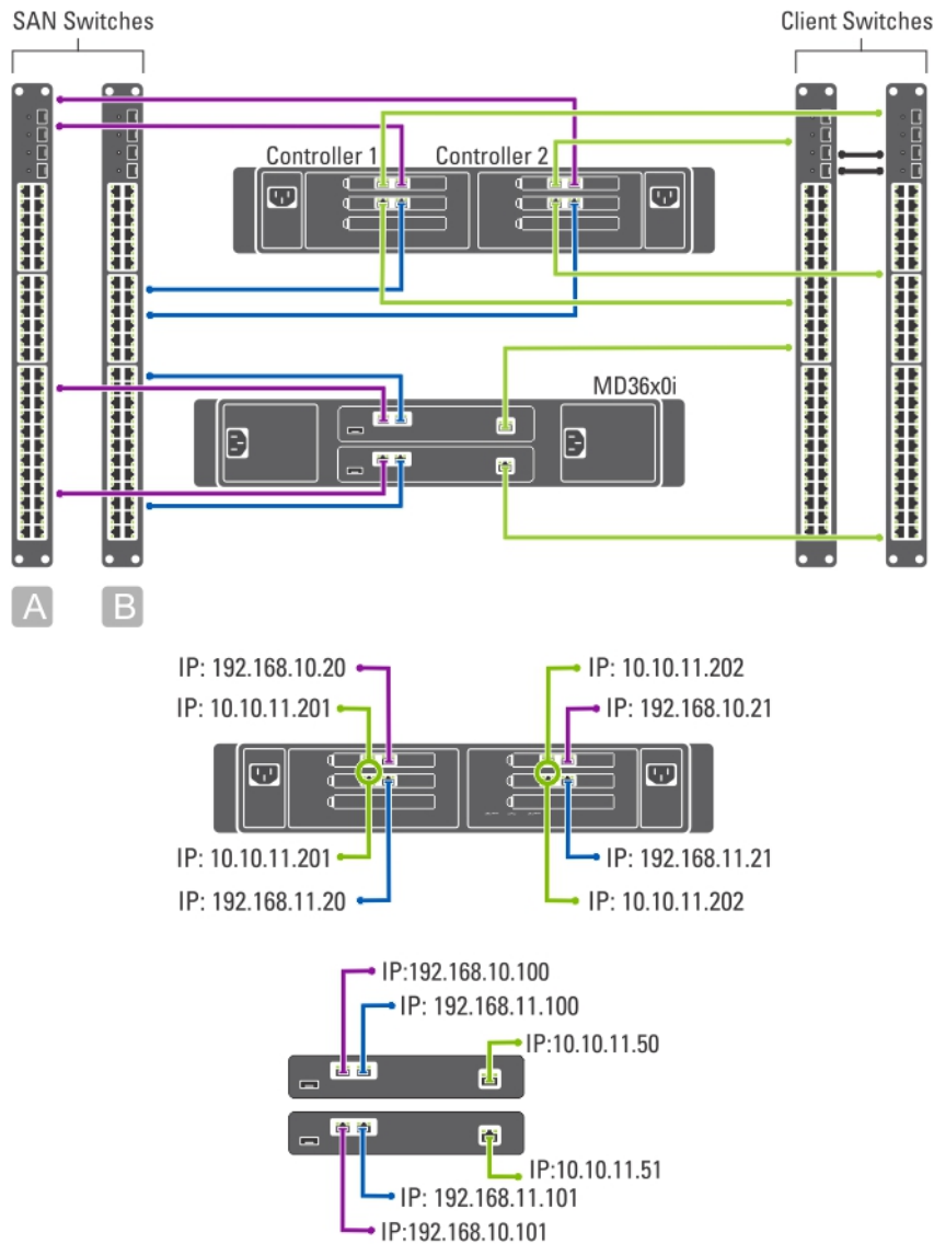
Figure 3. Solution SAN dédiée de l'option Disponibilité optimale
