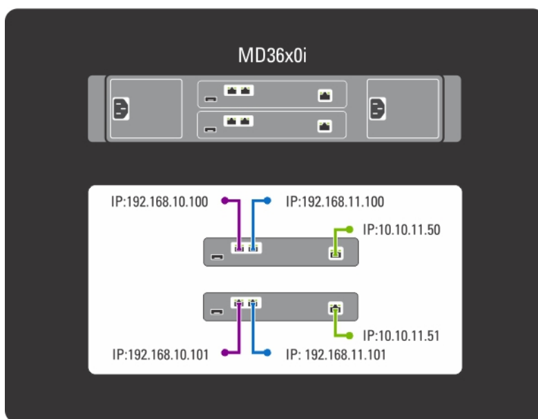
Figure 1. La topologie de commutateur MD
