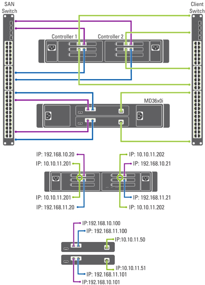
Figure 4. Solution SAN dédié de l'option non redondant
