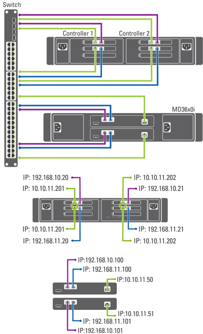
Figure 6. Option Non redondant tout en un
